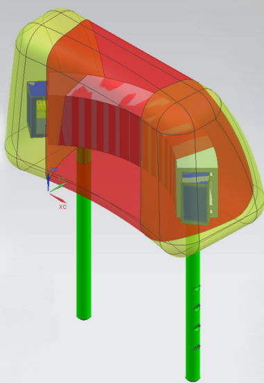
barevné znázornění hlavní částí opěrky hlavy před aktivací
